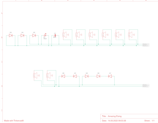
Görsel 7 (Piezo devresi tabanın ortasına yerleştirilecek)
